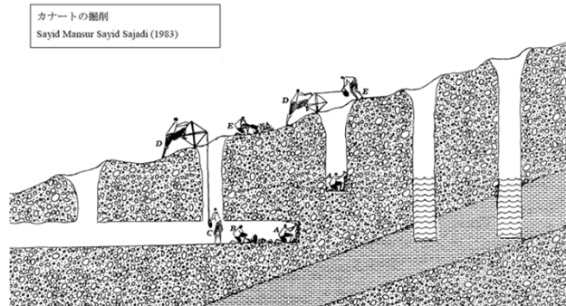
カナートの掘削方法
