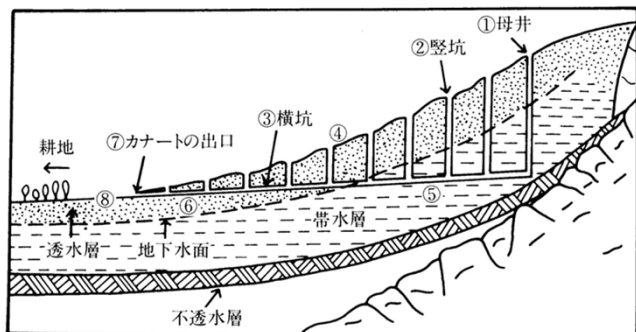
カナートの模式図
