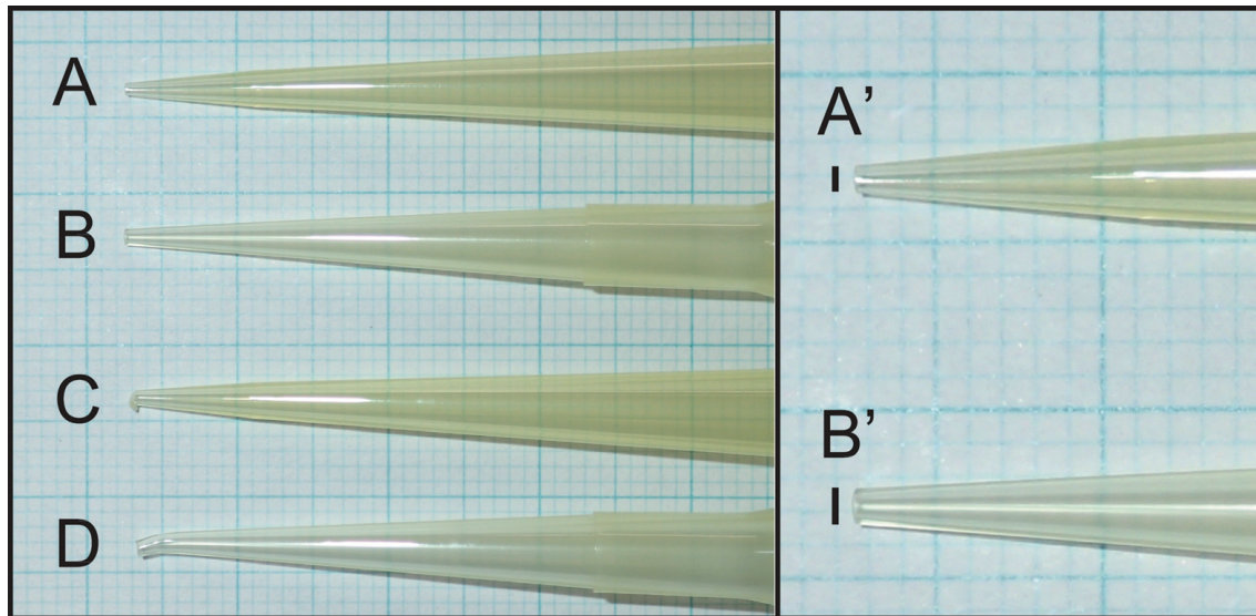
図 2. 破砕用マイクロピペットチップ，背景は 1 mm 方眼紙. A, 加工前のアイビス・ピペットチップ I-503Y (A'は A 先端部の拡大図); B, 加工前の他のピペットチップ (B'は B 先端部の拡大図); C, 加工後のアイビス・ピペットチップ I-503Y (先端が丸い破砕に適した形状に加工できた); D, 加工後の他のピペットチップ (先が折れ曲がった，破砕に不適な形状になりやすい). A'と B'における縦の黒色バーは各マイクロピペットチップの外径を示す. アイビス・ピペットチップ I-503Y はテーパ型となっており，外径は B よりも狭い.
